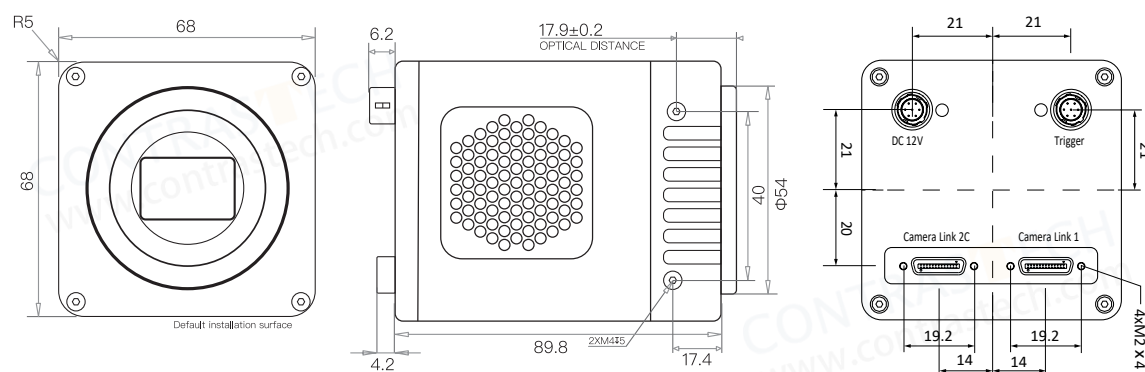
Dimensions C
