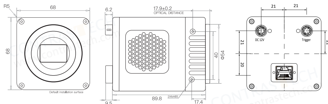
Dimensions B
