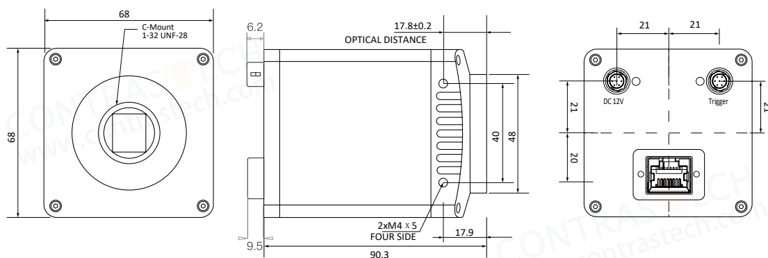
Dimensions B
