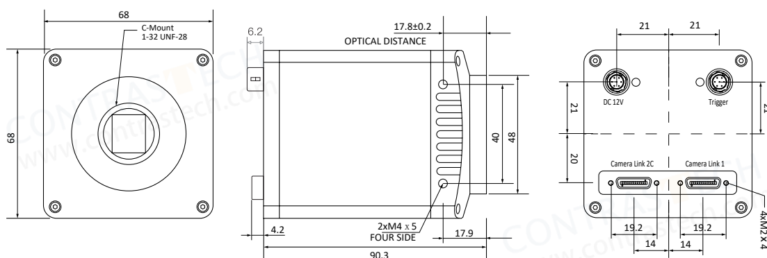
Dimensions C
