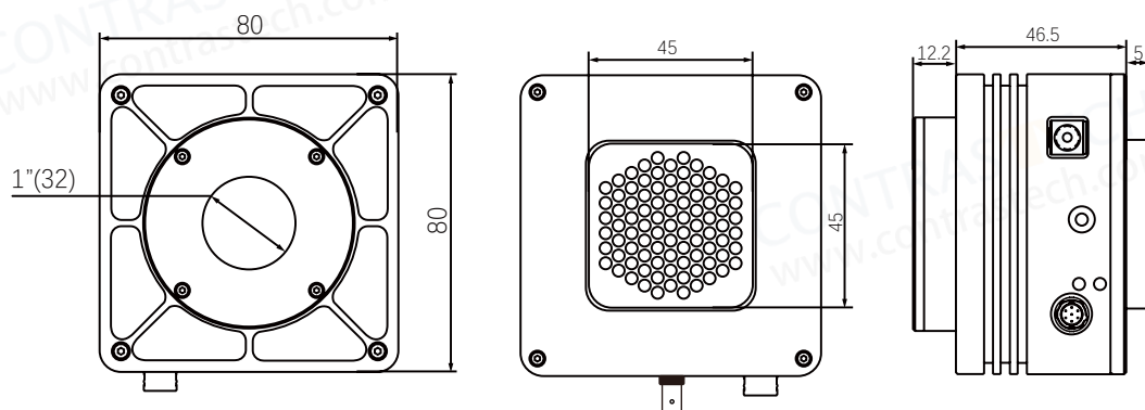
Dimensions C
