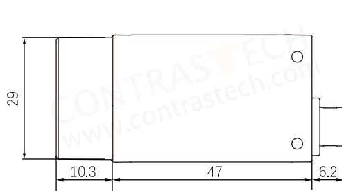
Dimensions D
