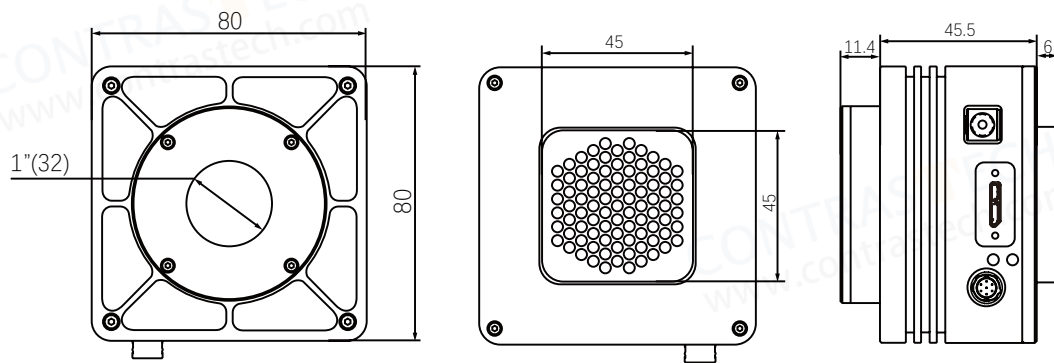
Dimensions B
